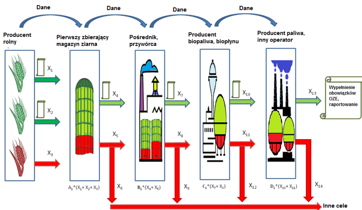
Rys. 1 Schemat bilansu masy Systemu KZR INiG-PIB
